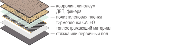
Рис. Схема монтажа теплого пола CALEO под ламинат, ковролин, линолеум
